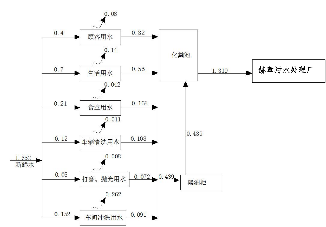
图2-1 项目建成后水平衡图 (m³/d)
